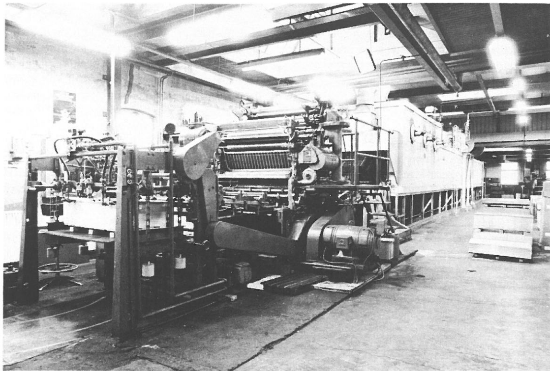
De blikdrukpers van het type Mailander met moffeloven. Aan de achterzijde is de laklijn zichtbaar. Deze foto werd ruim een jaar voor de sluiting gemaakt, in 1988. De foto is deel van een serie die fotograaf Niek Bavelaar maakte toen bekend werd dat Van Leer de poorten in Leiden zou sluiten. De directie stelde als voorwaarde dat de foto's pas na sluiting van de fabriek gepubliceerd zouden worden. Oliemaatschappij Shell was in die jaren de voornaamste klant en Van Leer vreesde 'ongewenste aandacht' van actiegroepen als haar activiteiten aandacht zouden trekken. (foto Niek Bavelaar)
